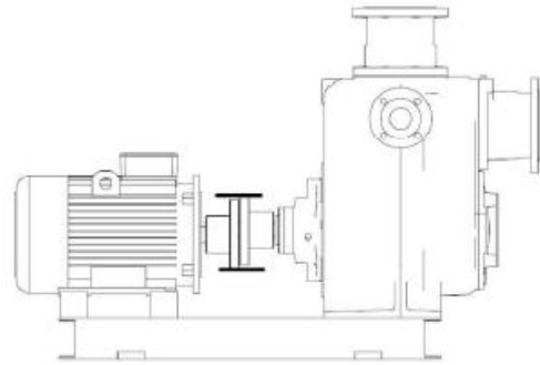
(Figuur 3-4) Fout bij parallel in verticaal vlak
