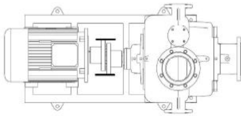
(Figuur 3-3) Fout bij parallel in horizontaal vlak
